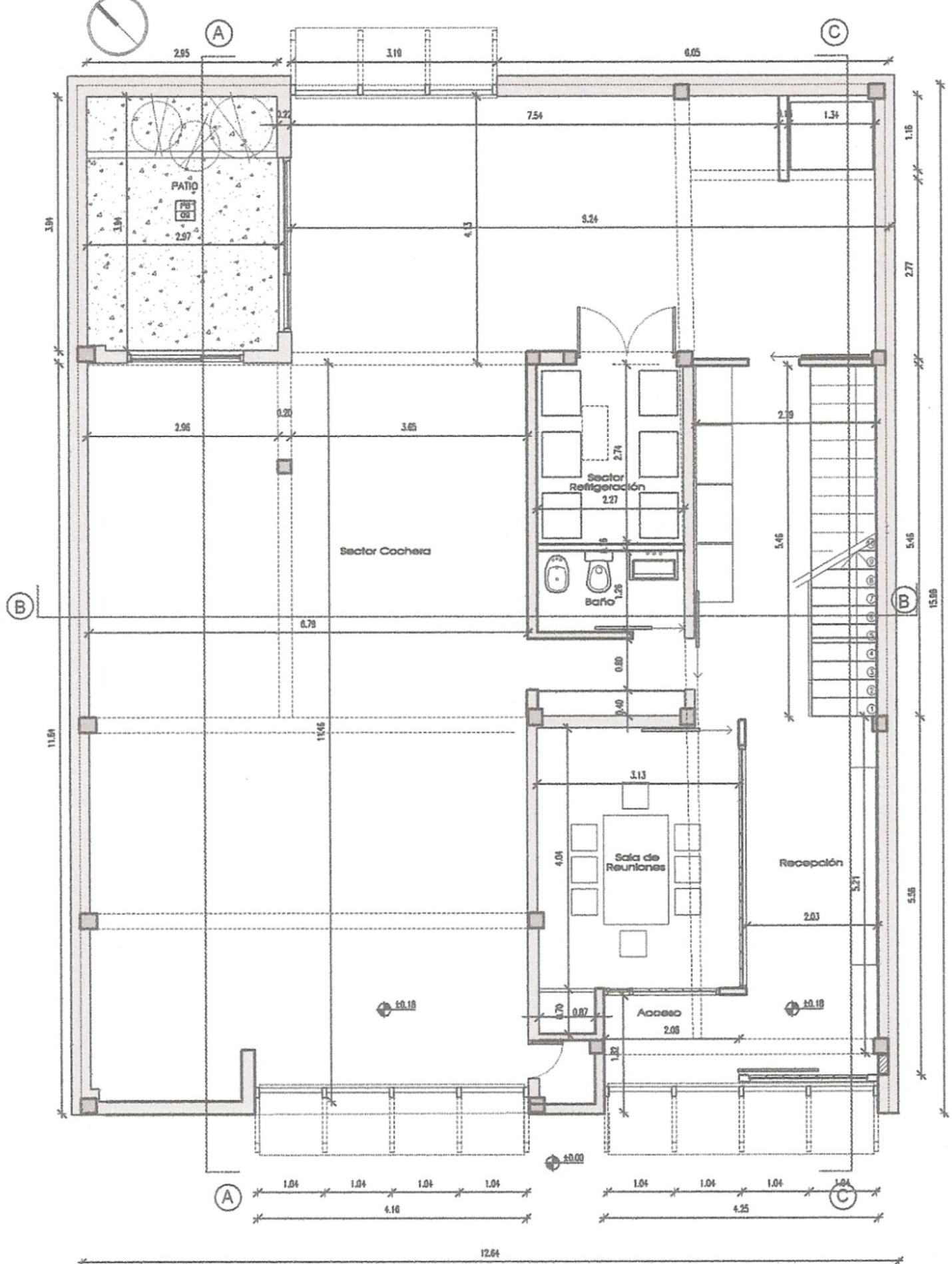
Planta Baja
